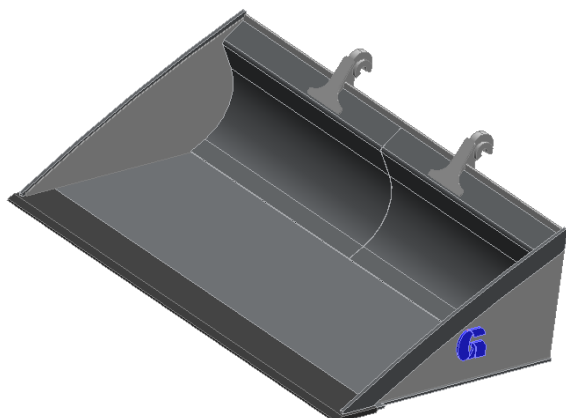
Frontplanerskopa 2700 mm. Med L90
